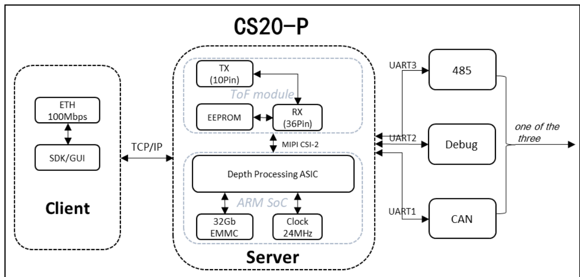
Figure 2-2. CS20-P 以太网深度相机系统框图
