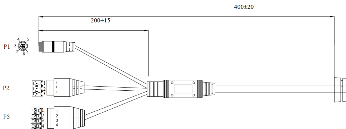
Figure 3-1. CS20-P 尾线示意图
