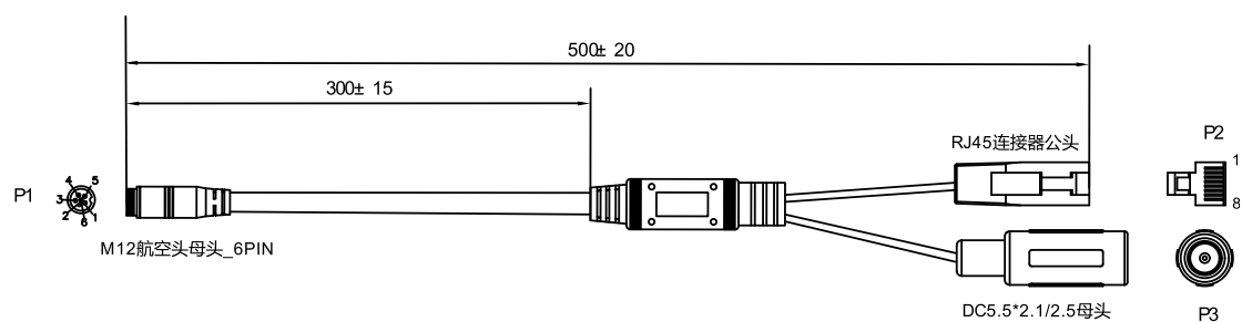
Figure 3-2. CS20-P 转接线示意图
