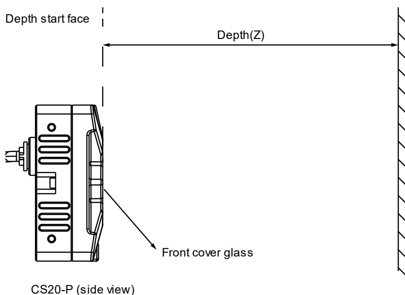
Figure 4-1 CS20-P 评测起点
