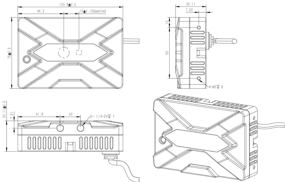
Figure 5-1 CS20-P 以太网深度相机结构示意图
